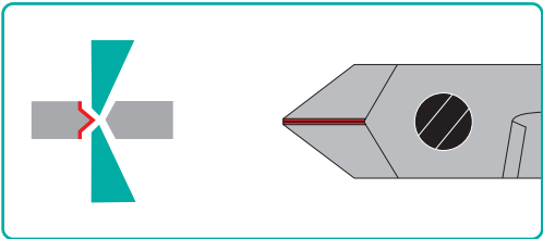
Mini bevel
